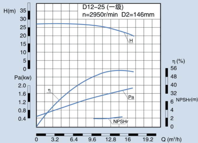
CMB 12-25 性能表
