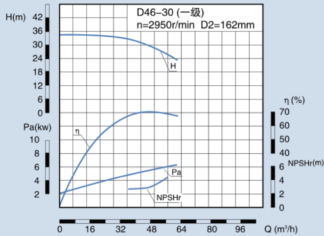
CMB 46-30 性能表
