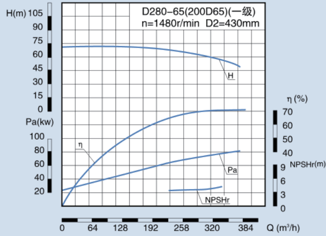
CMB 280-65(200 65) 性能表
