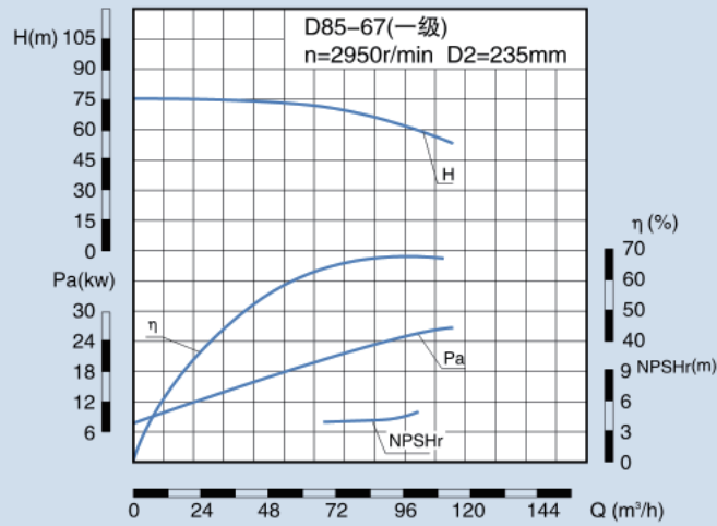
CMB 85-67 性能表
